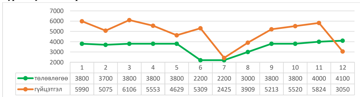
График5. Уураар түгээсэн дулааны эрчим хүч
